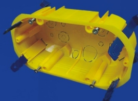
KSC 11-107 Электроустановочная коробка для гипсокартона и полых стен H-50
